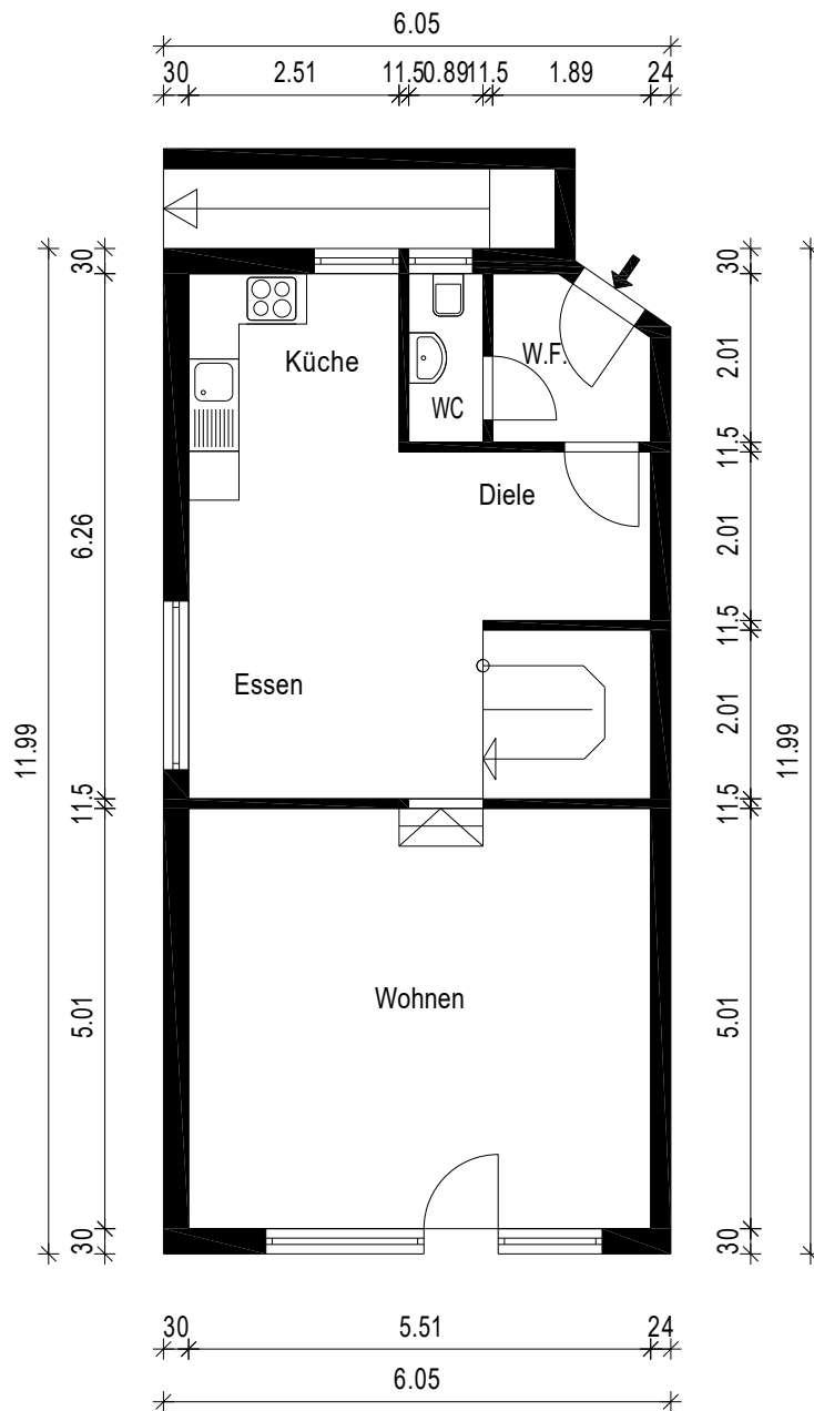
Erdgeschoss
