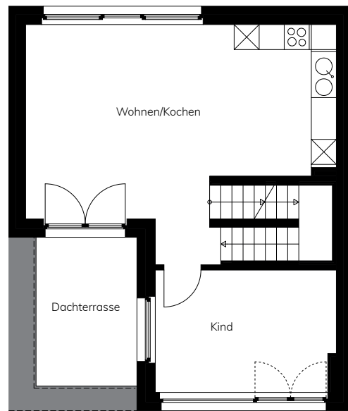
OBERGEHOSS
