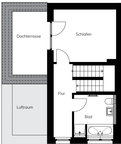
DACHGESCHOSS
