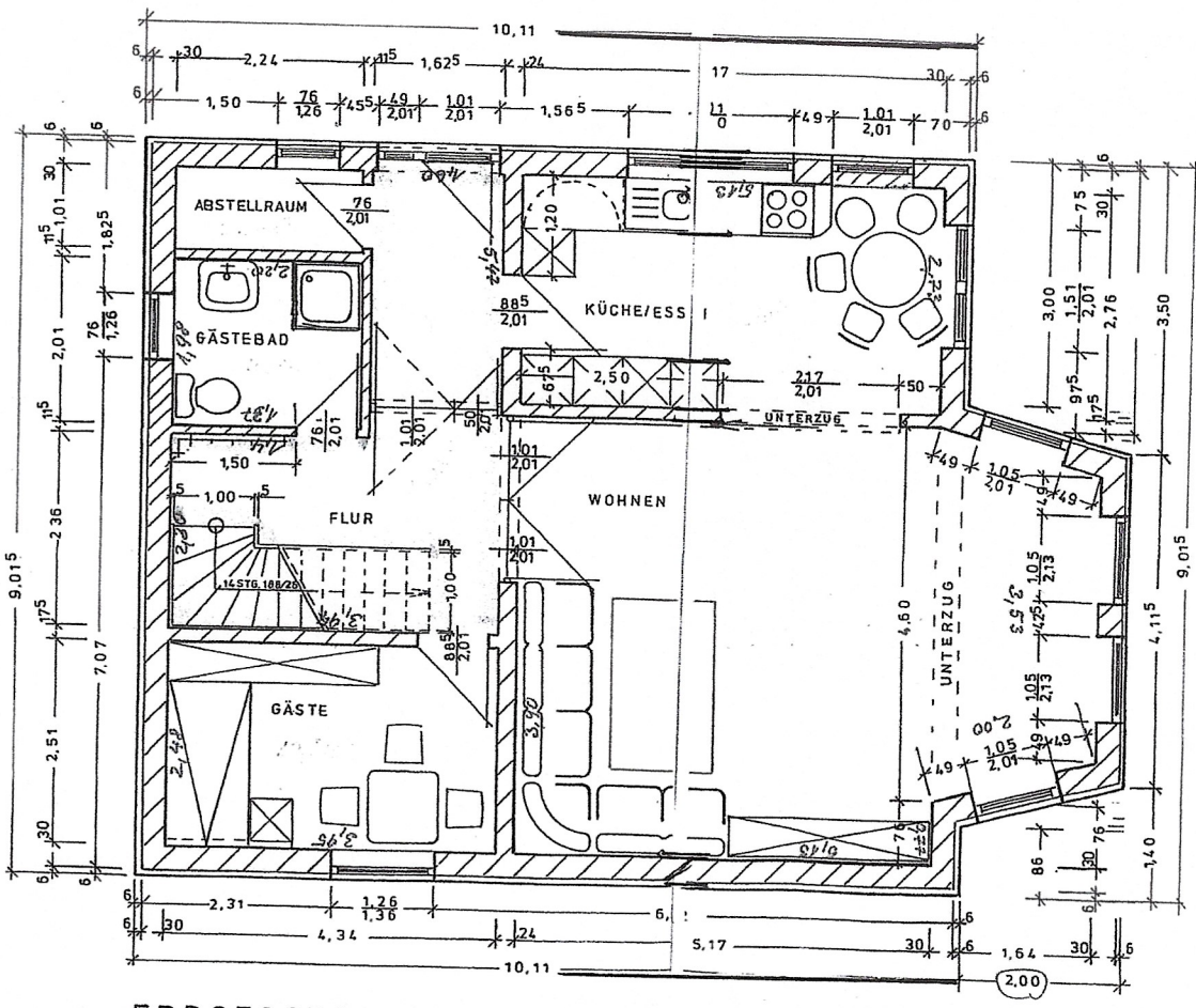
ERDGESCHOSSGRUNDRISS M1:100
