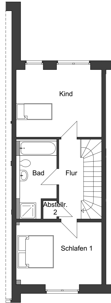
Grundriss 1.OG
