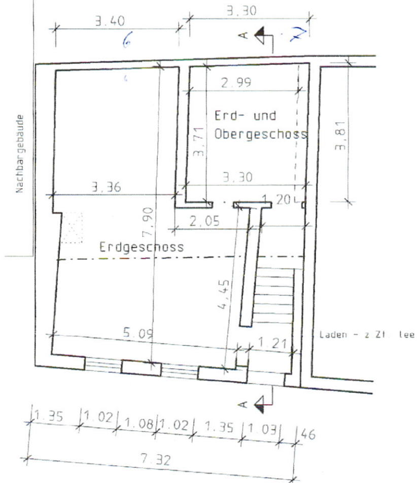
GRUNDRISS - VORHANDEN
