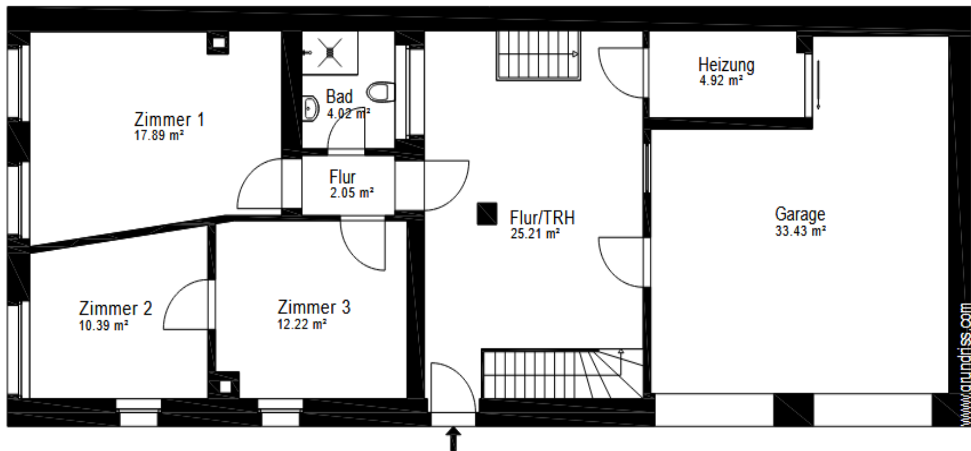
Grundriss EG
