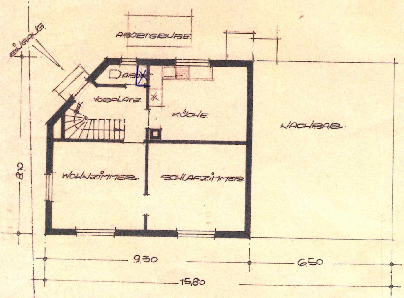
Erdgeschoss
