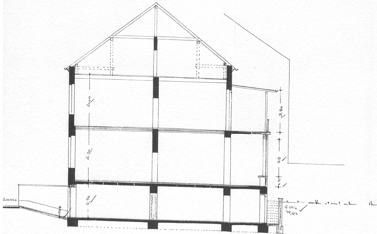
QUERSCHNITT DURCH DAS VORGERÄUS
