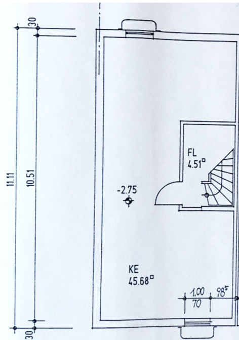
KELLERGESCHOSS 50.19 M 2 HAUSTYP CK
