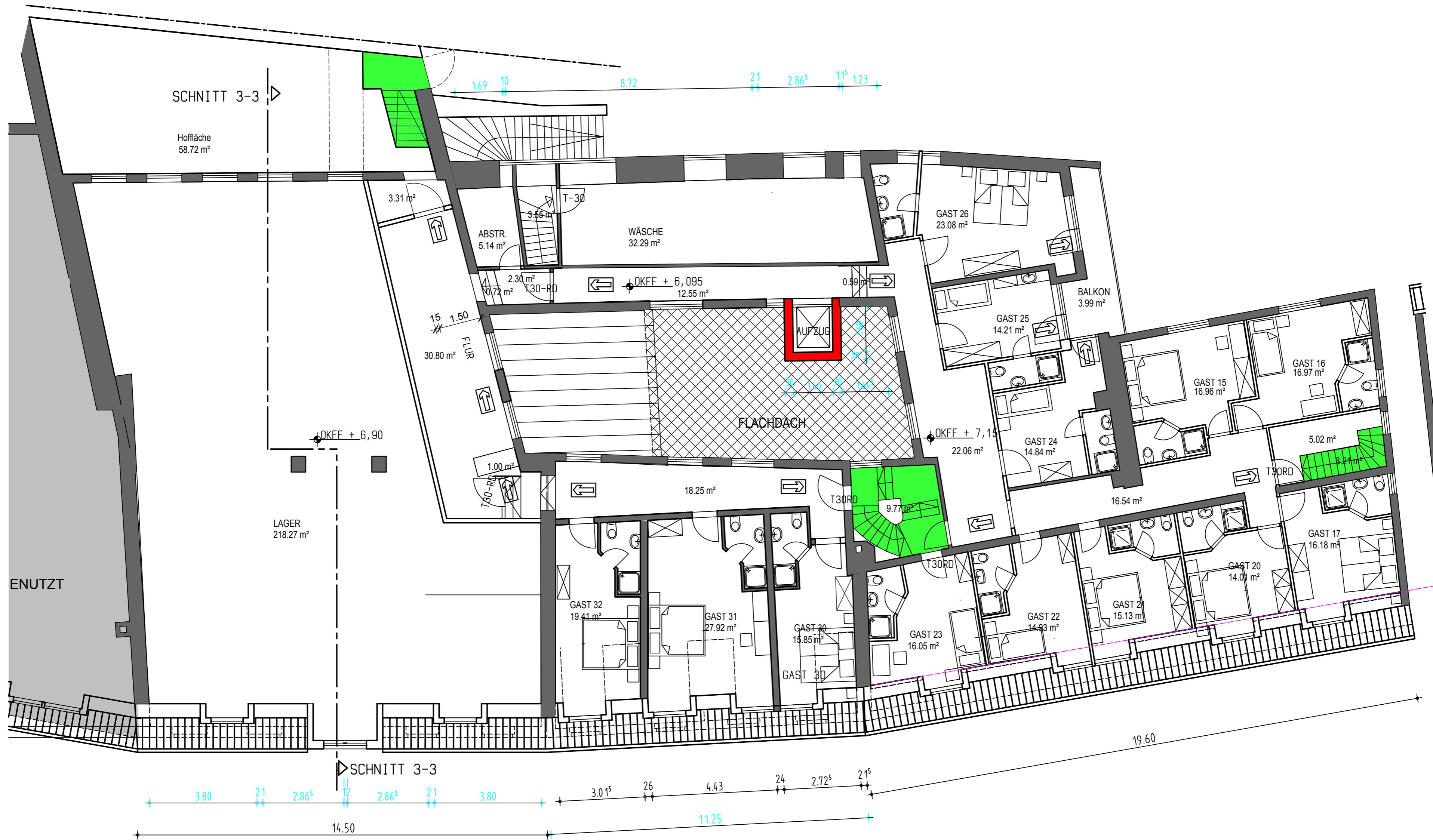
GRUNDRISS 2.OBERGESCHOSS 1.DACHGESCHOSS
