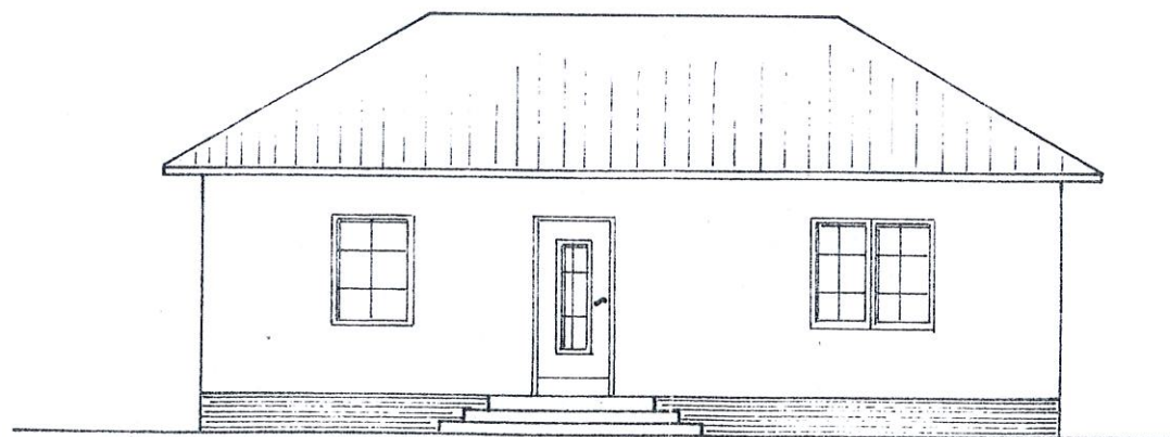
Nordansicht
