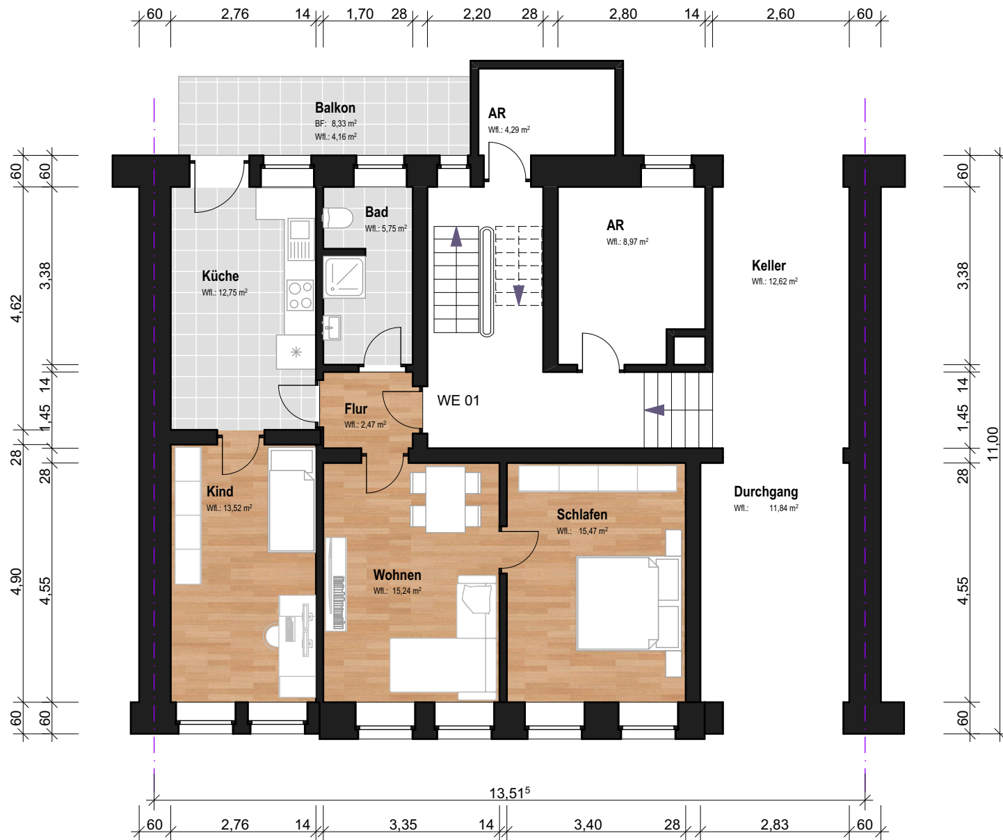
Grundriss Erdgeschoss
