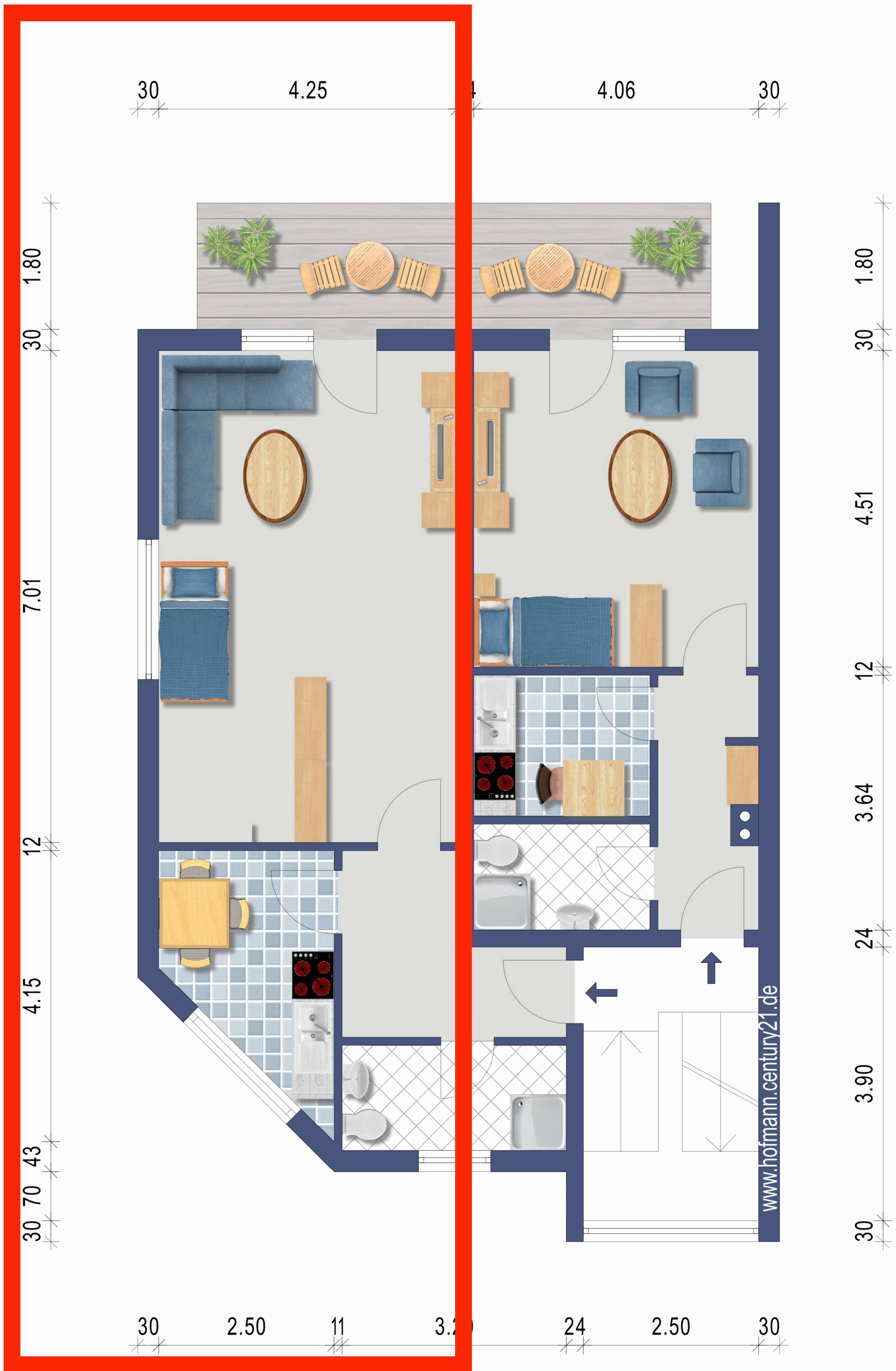
1.Obergeschoss
