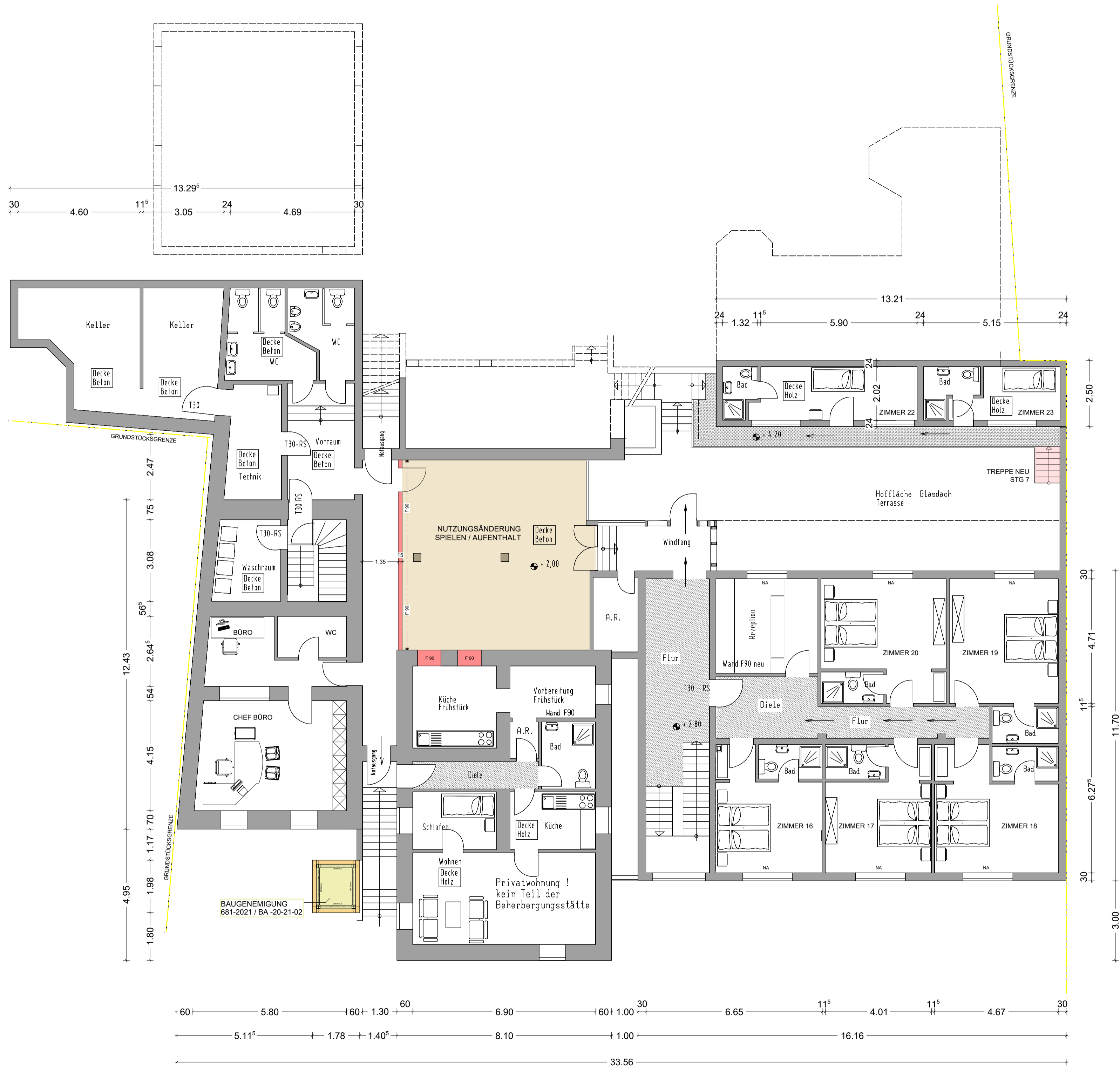
OBERGESCHOSS I
