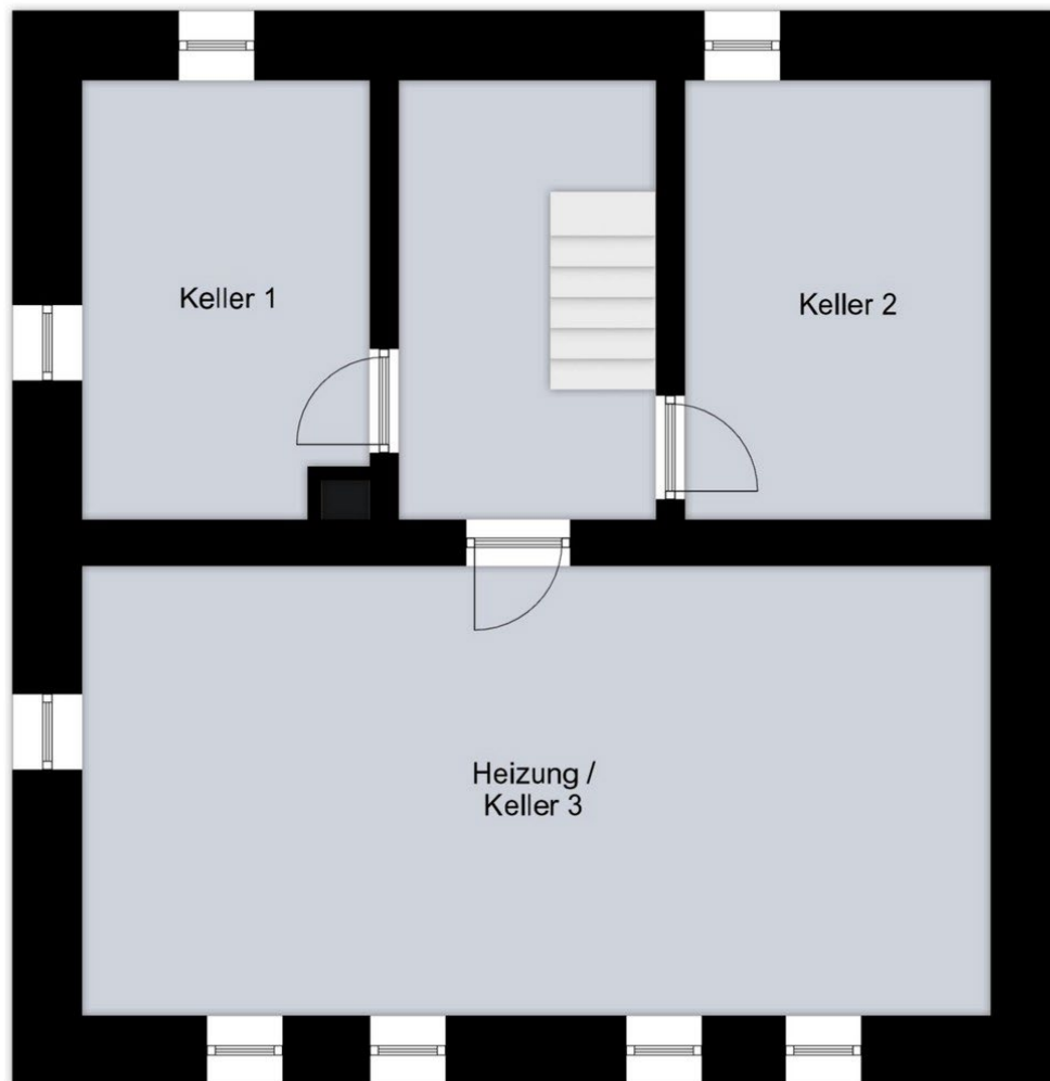
Haus 1 - Kellergeschoss
