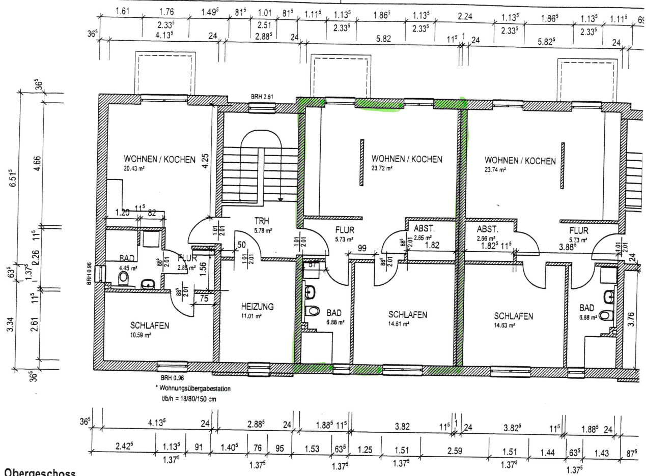
Obergeschoss
