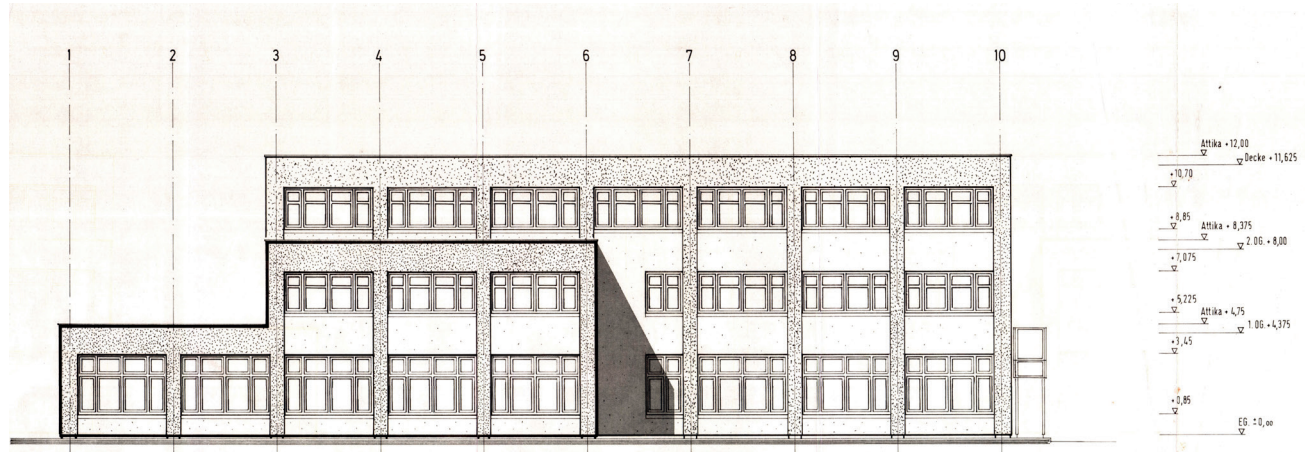
OST - ANSICHT
