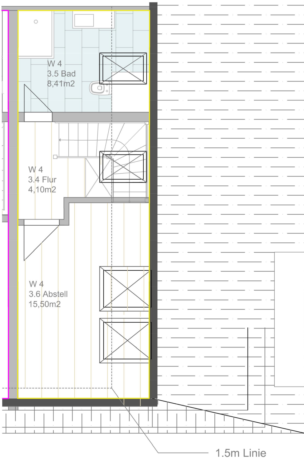
Wohnung 4 Grundriss Spitzboden M 1:50
