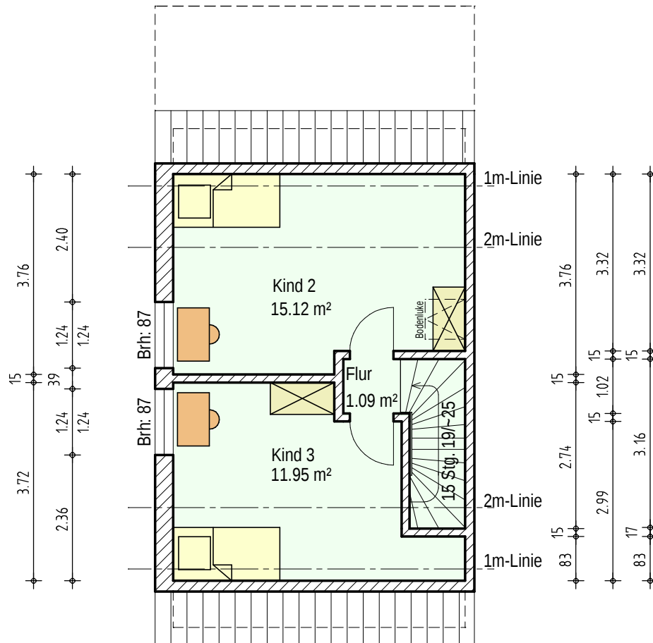
Möblierungsvorschlag
