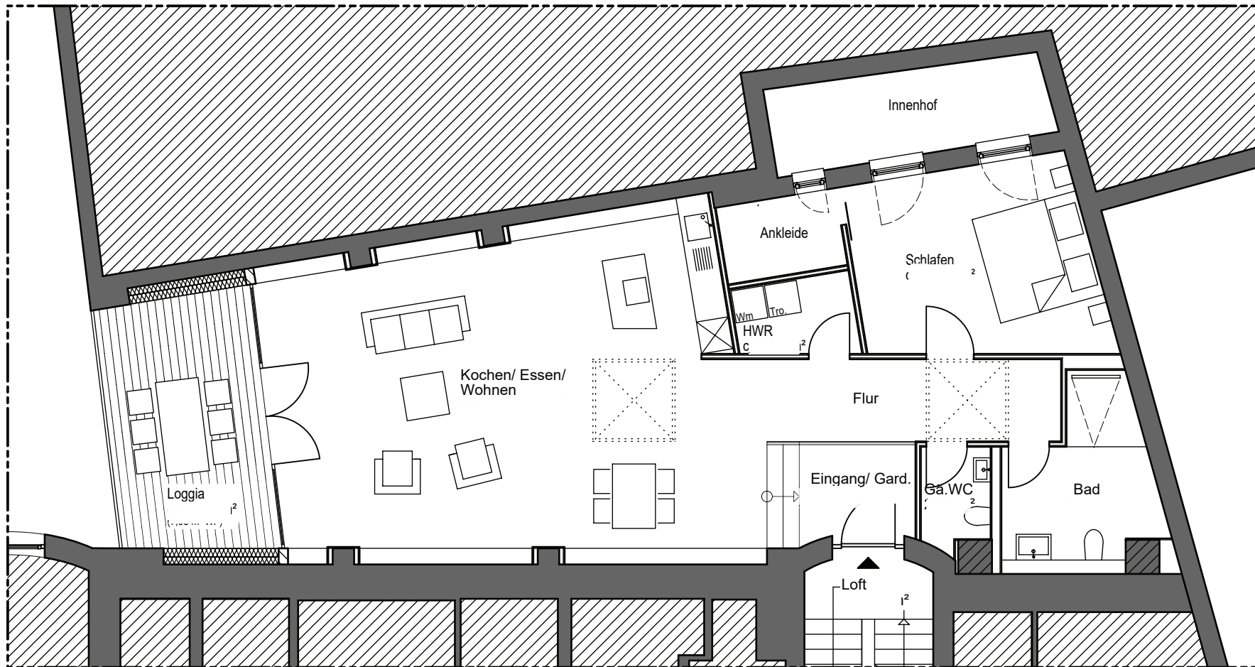
M 1:100
