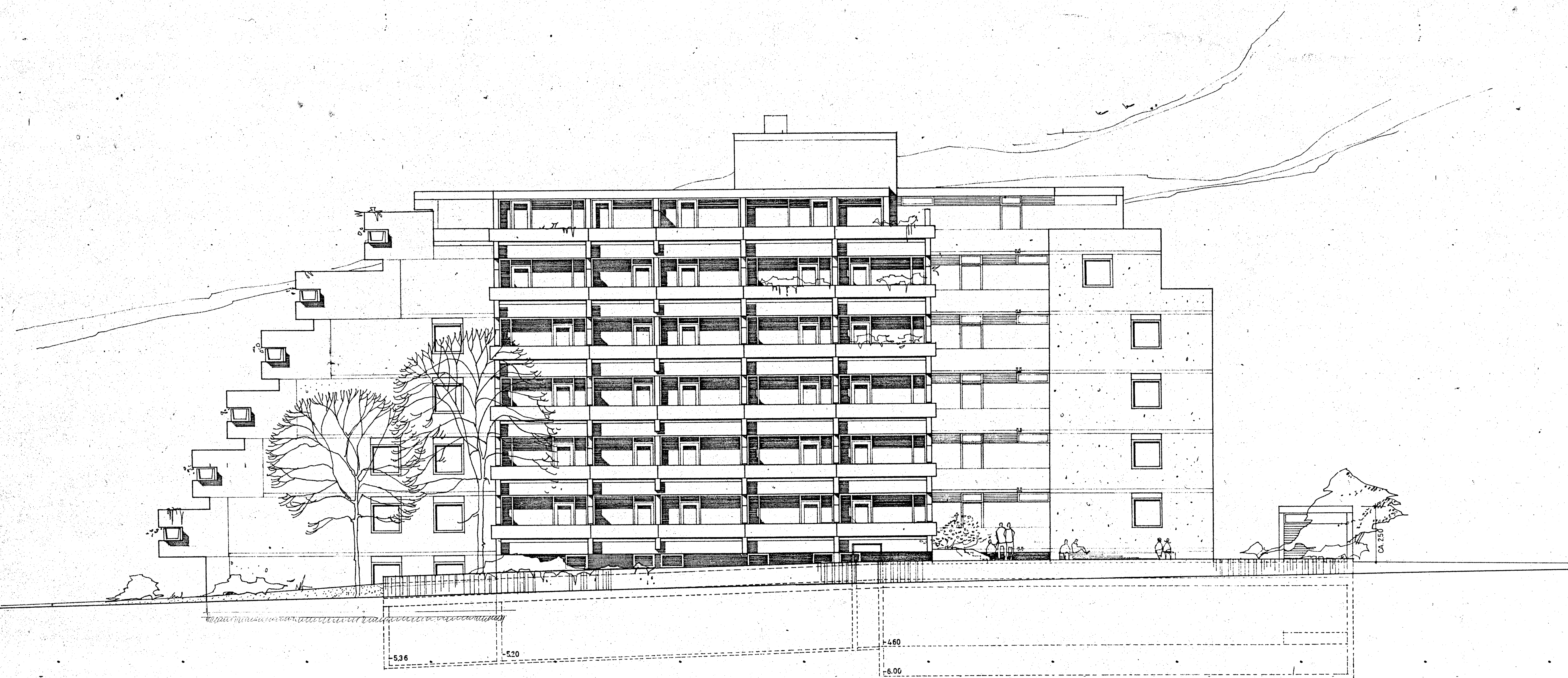
ANSICHT OSTEN
