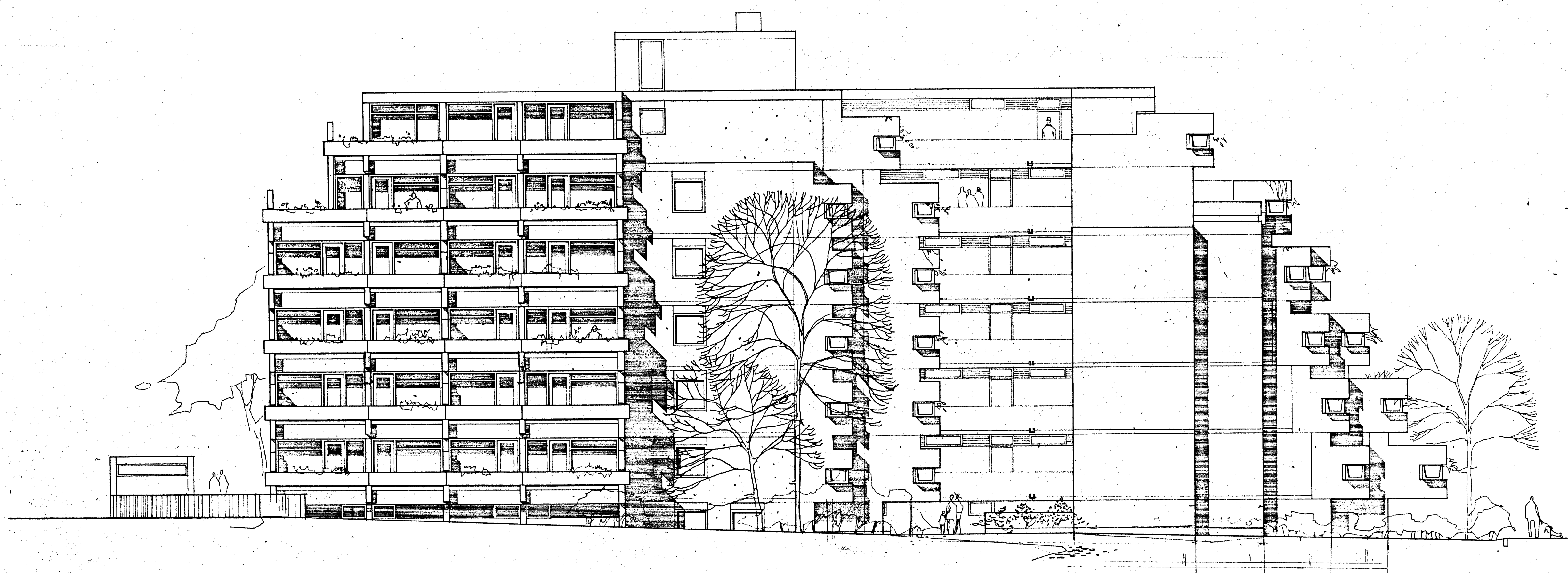
ANSICHT WESTEN
