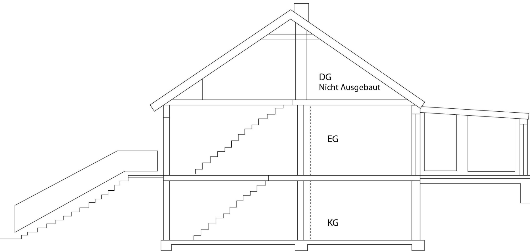
Schnitt A-A
