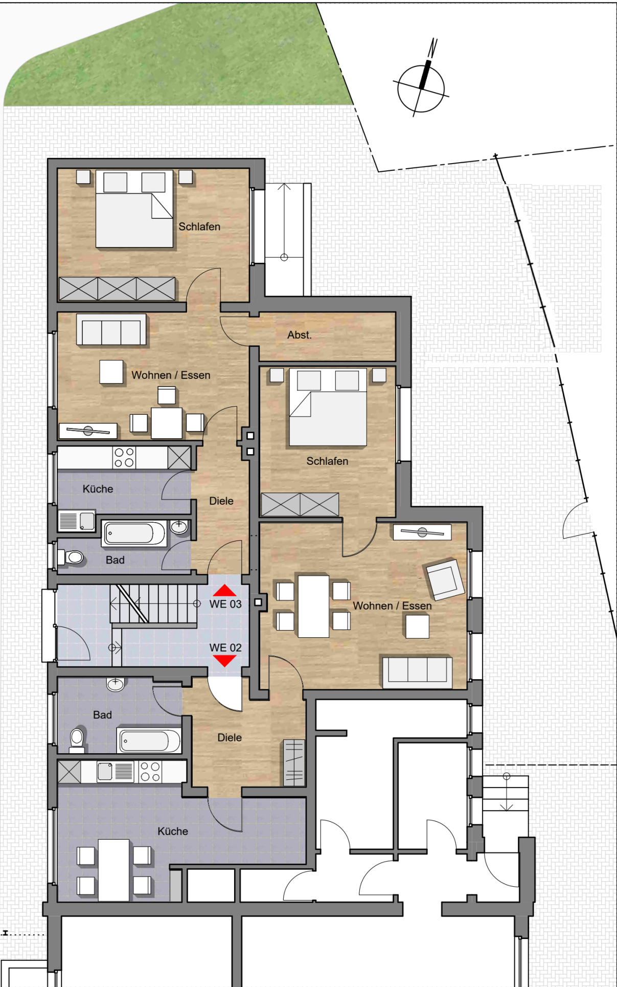
Grundriss Wohnungen 02 & 03
