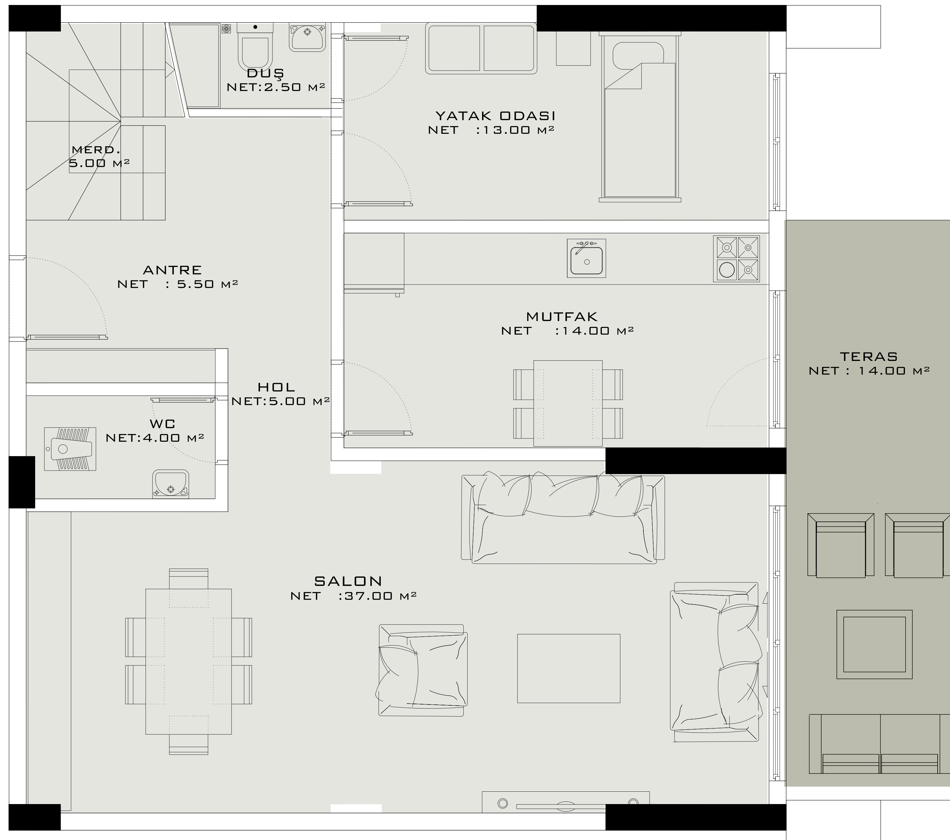
GİRİŞ KAT PLANI
