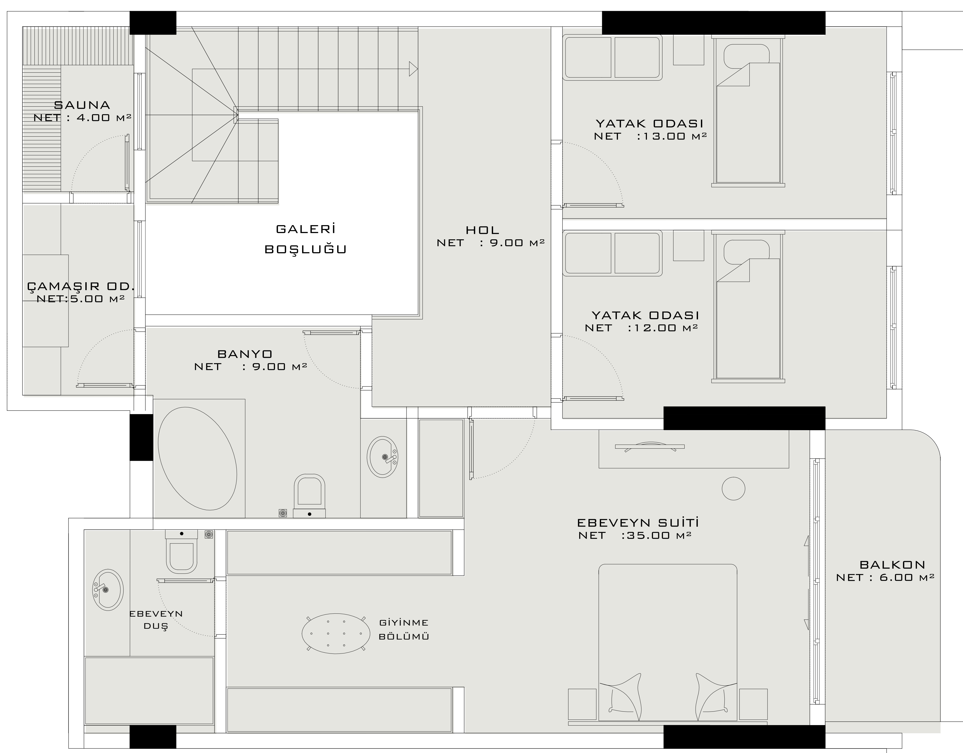
ÜST KAT PLANI
