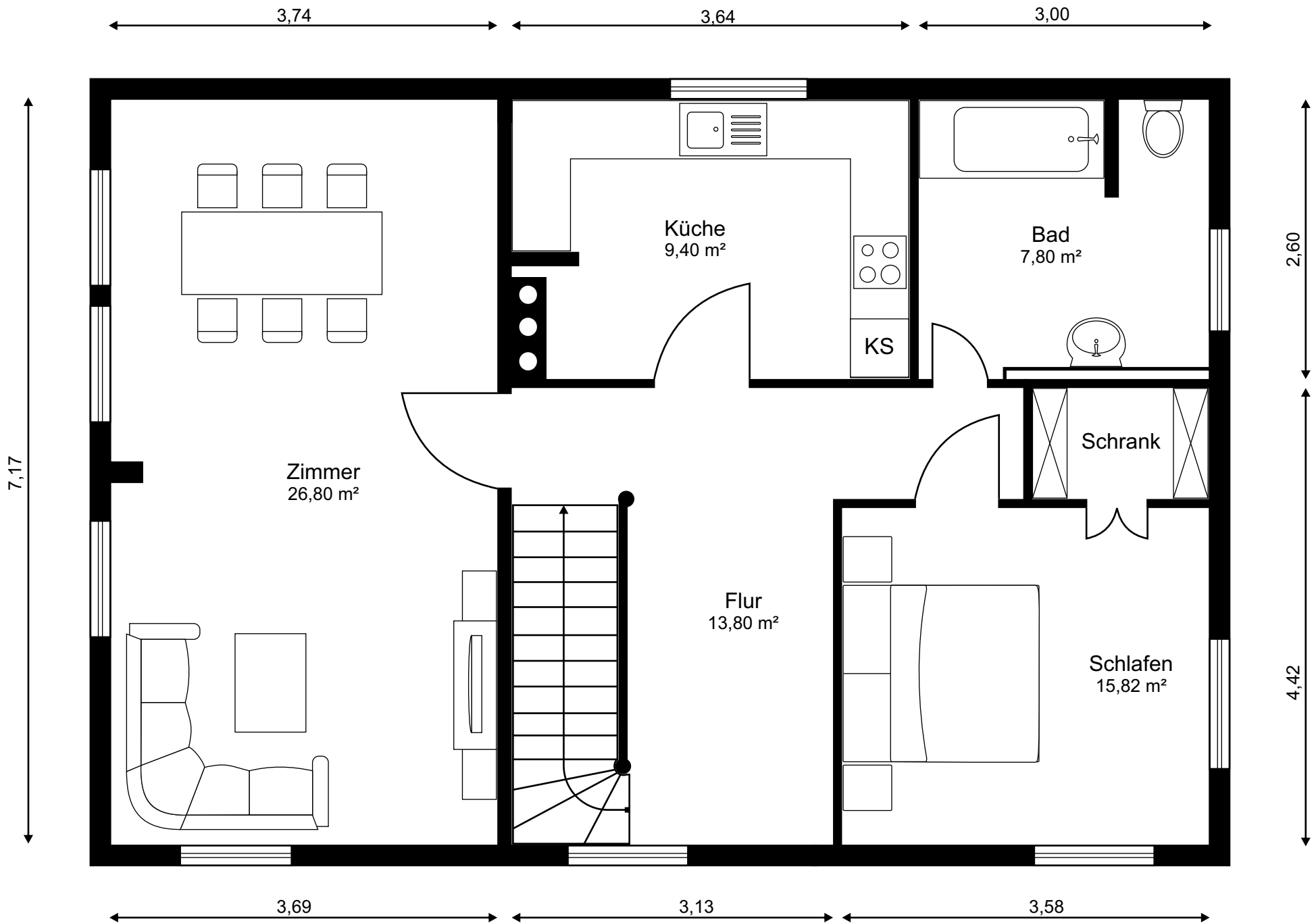
Obergeschoss
