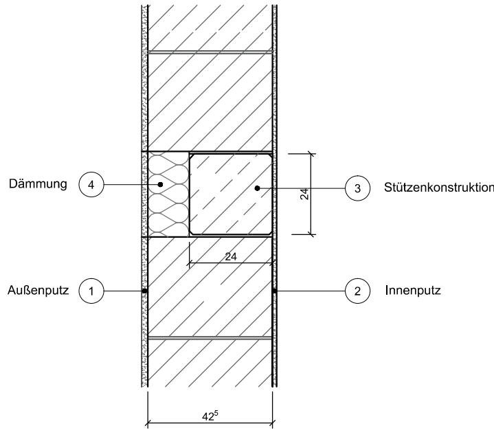
Detail Stütze in der Wand M 1:15
