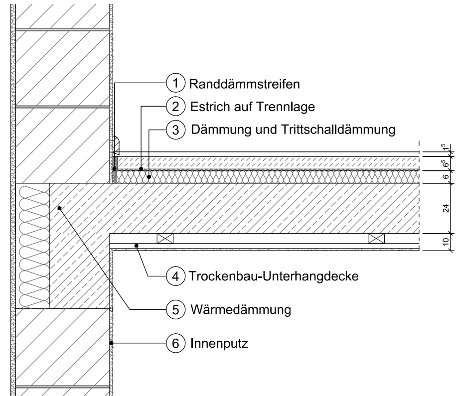
Detail Einbindende Decke in Außenwand M 1:15
