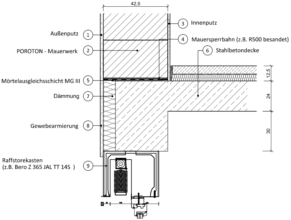
Detail Sturzbereich mit Ziegel-Raffstorekasten M 1:15
