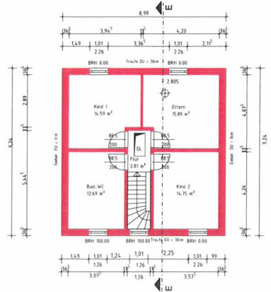
Obergeschoß
