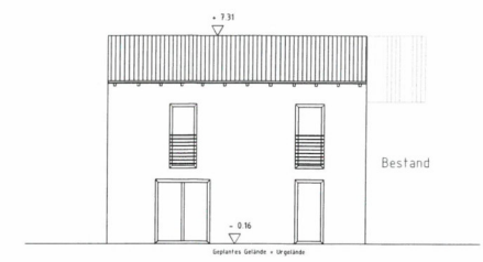
Nord-Ansicht
