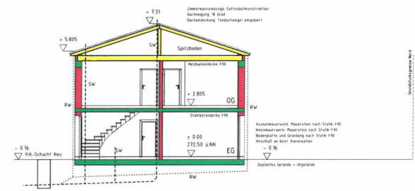
SCHNITT E-E
