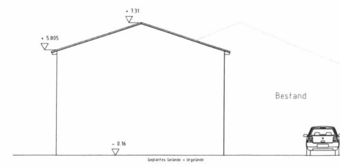
Ost-Ansicht
