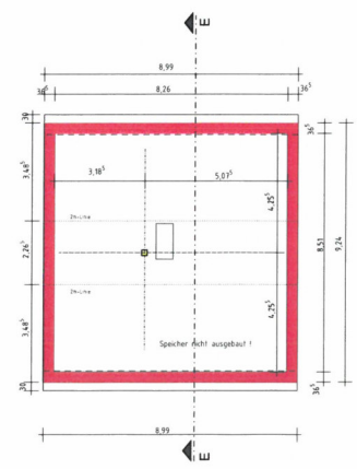
Spitzboden
