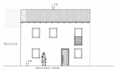
Süd-Ansicht
