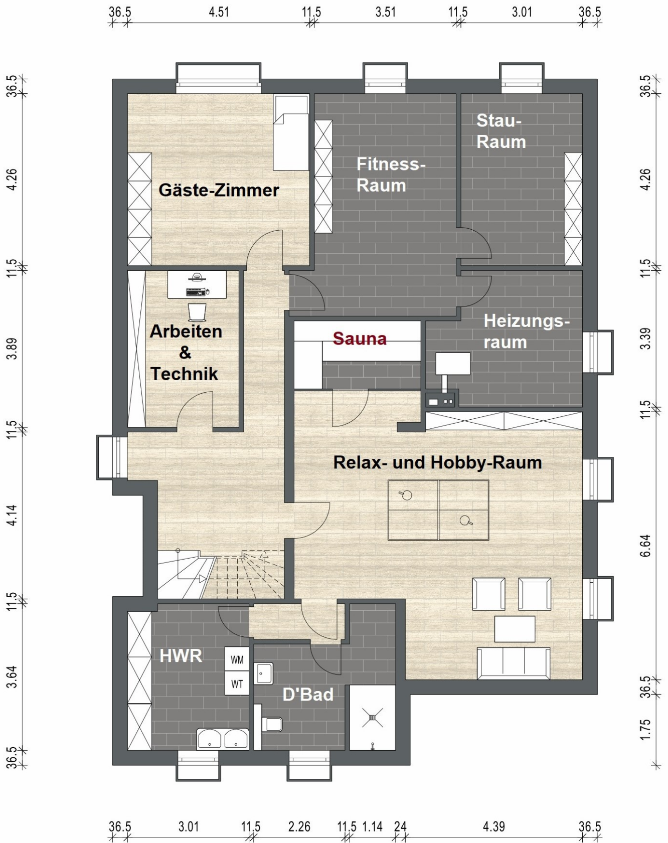
Kellergeschoss
