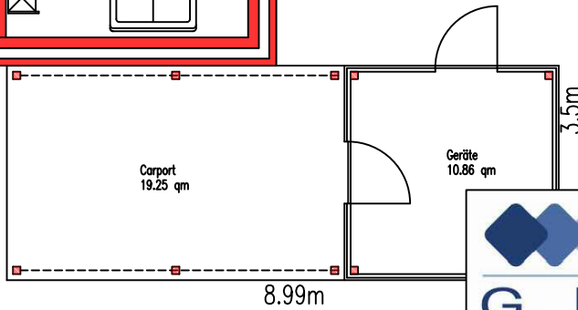
Erdgeschoss
