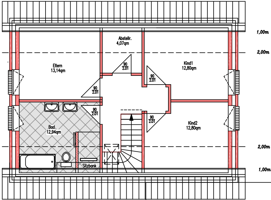
Dachgeschoss
