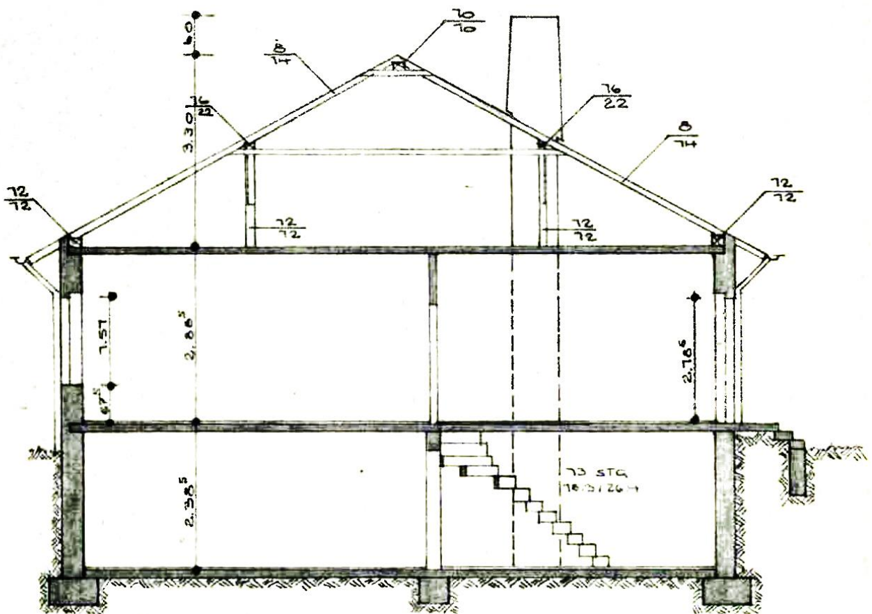
SCHNITT A-B
