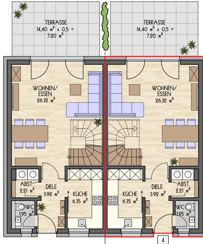
GRUNDRISS ERDGESCHOSS WOHNUNG 4
