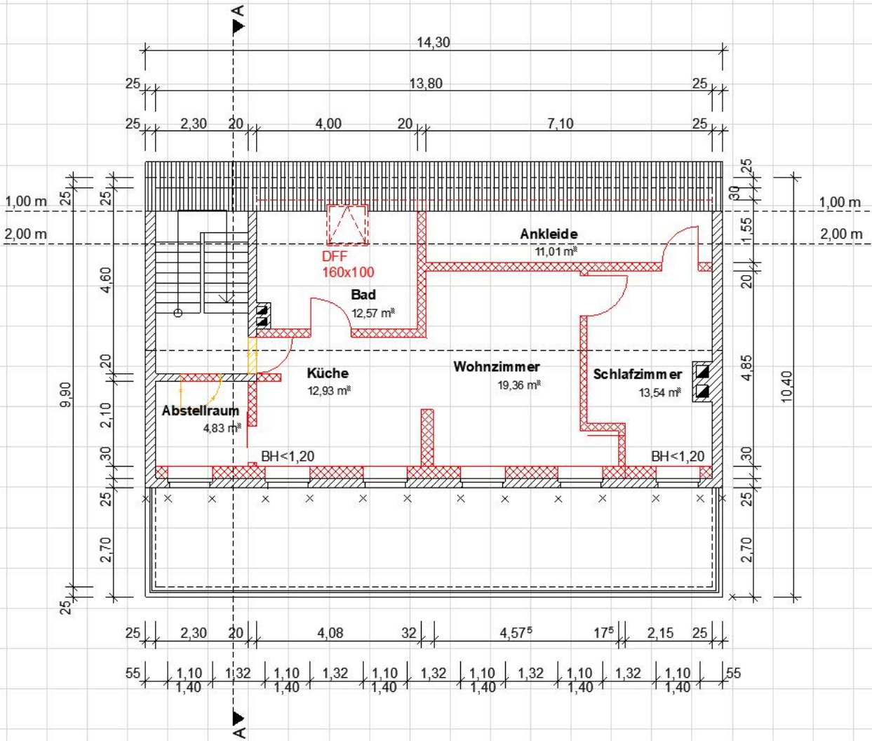
Grundriss Dachgeschoss
