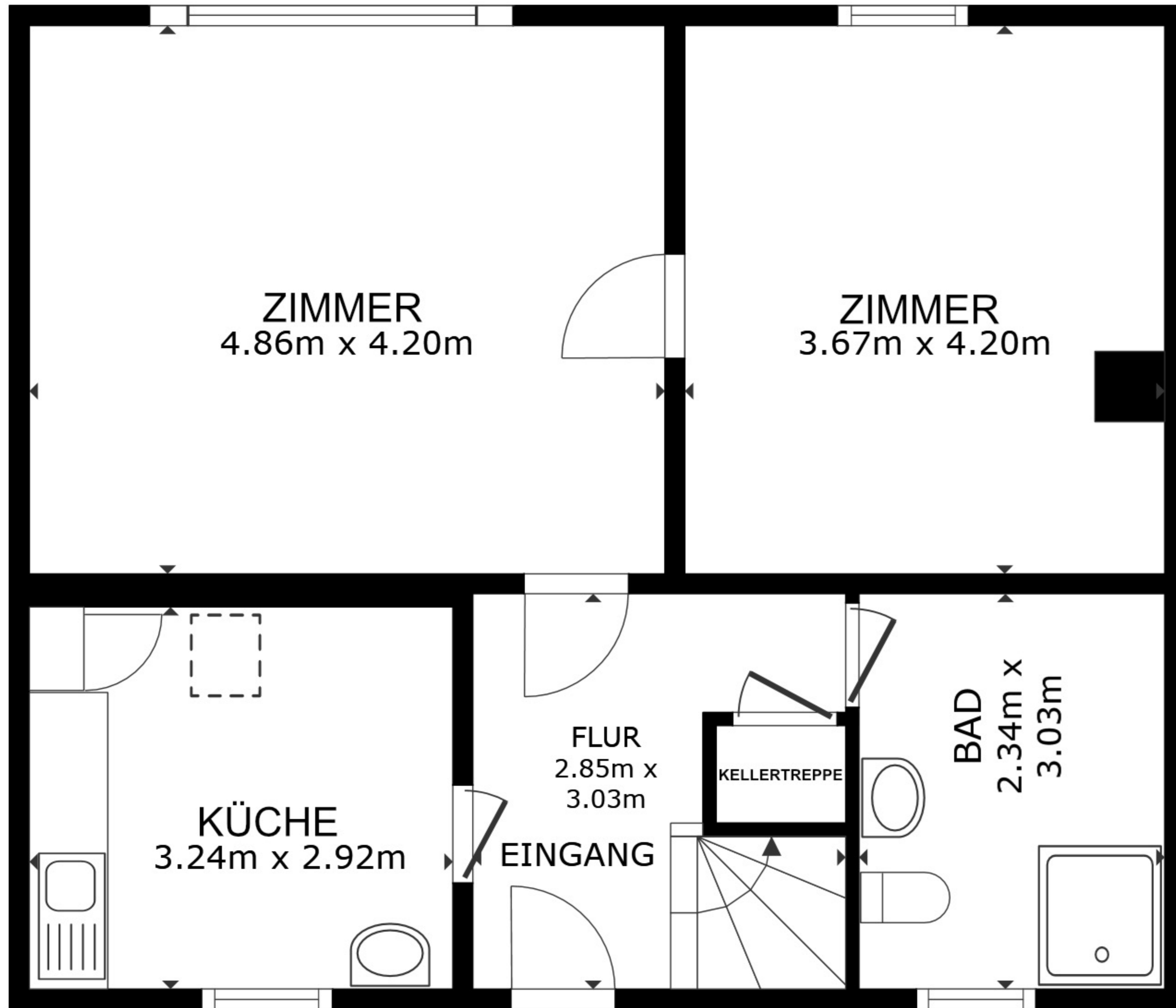
STOCKWERK 1
