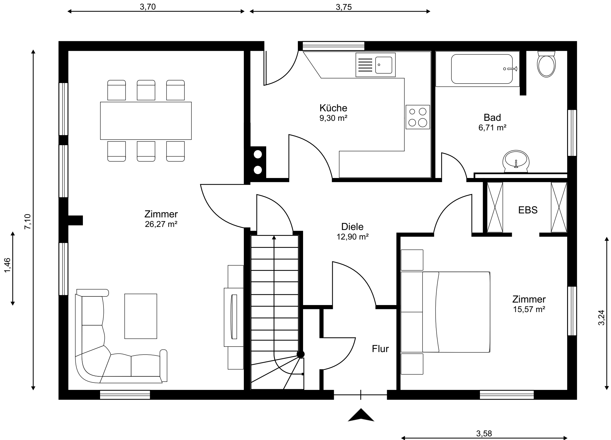
Erdgeschoss
