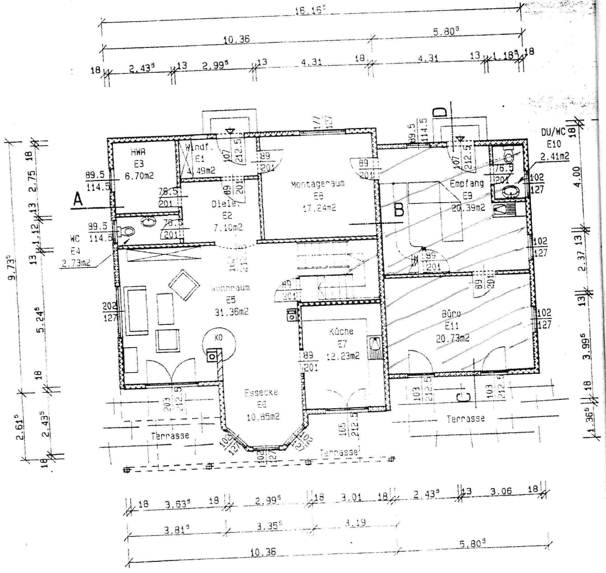
Erdgeschoss
