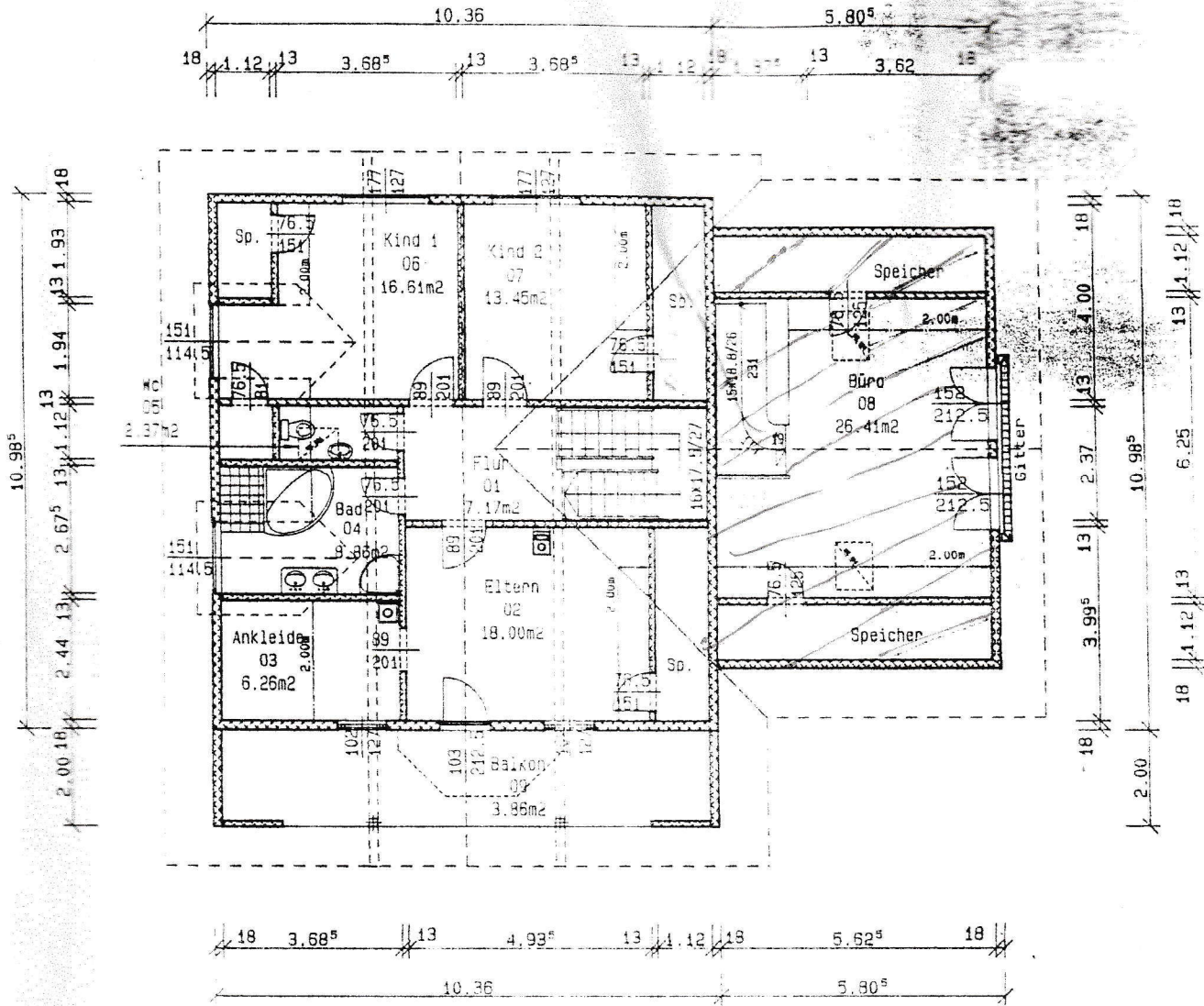
Obergeschoss
