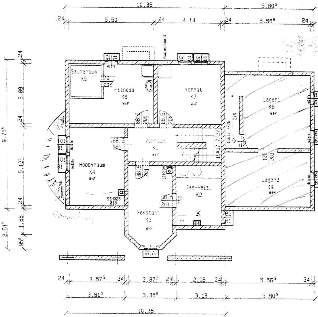
Kellergeschoss
