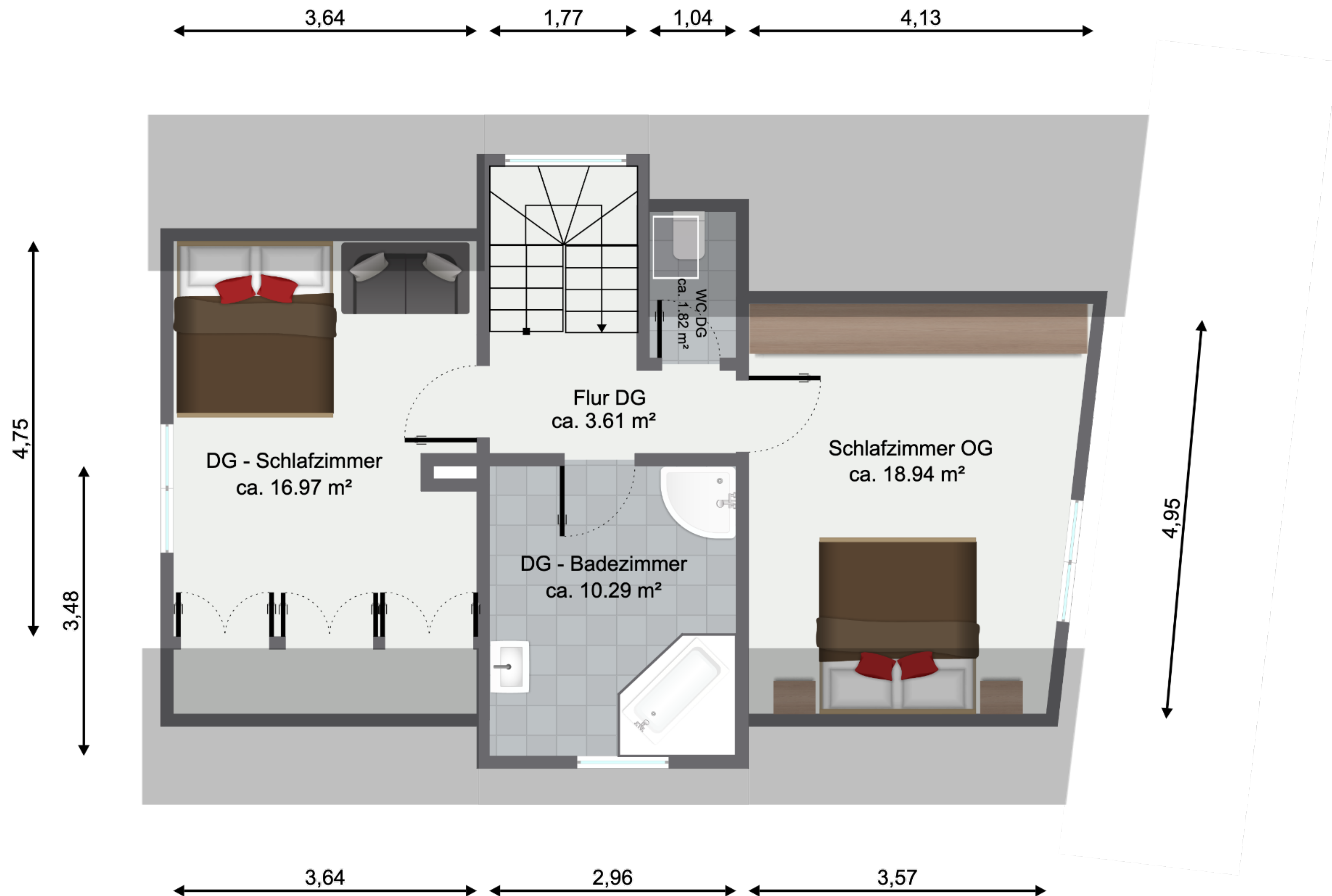
Dachgeschoss
