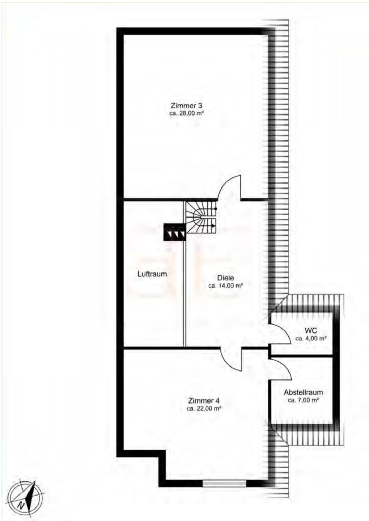
Grundriss – obere Ebene
