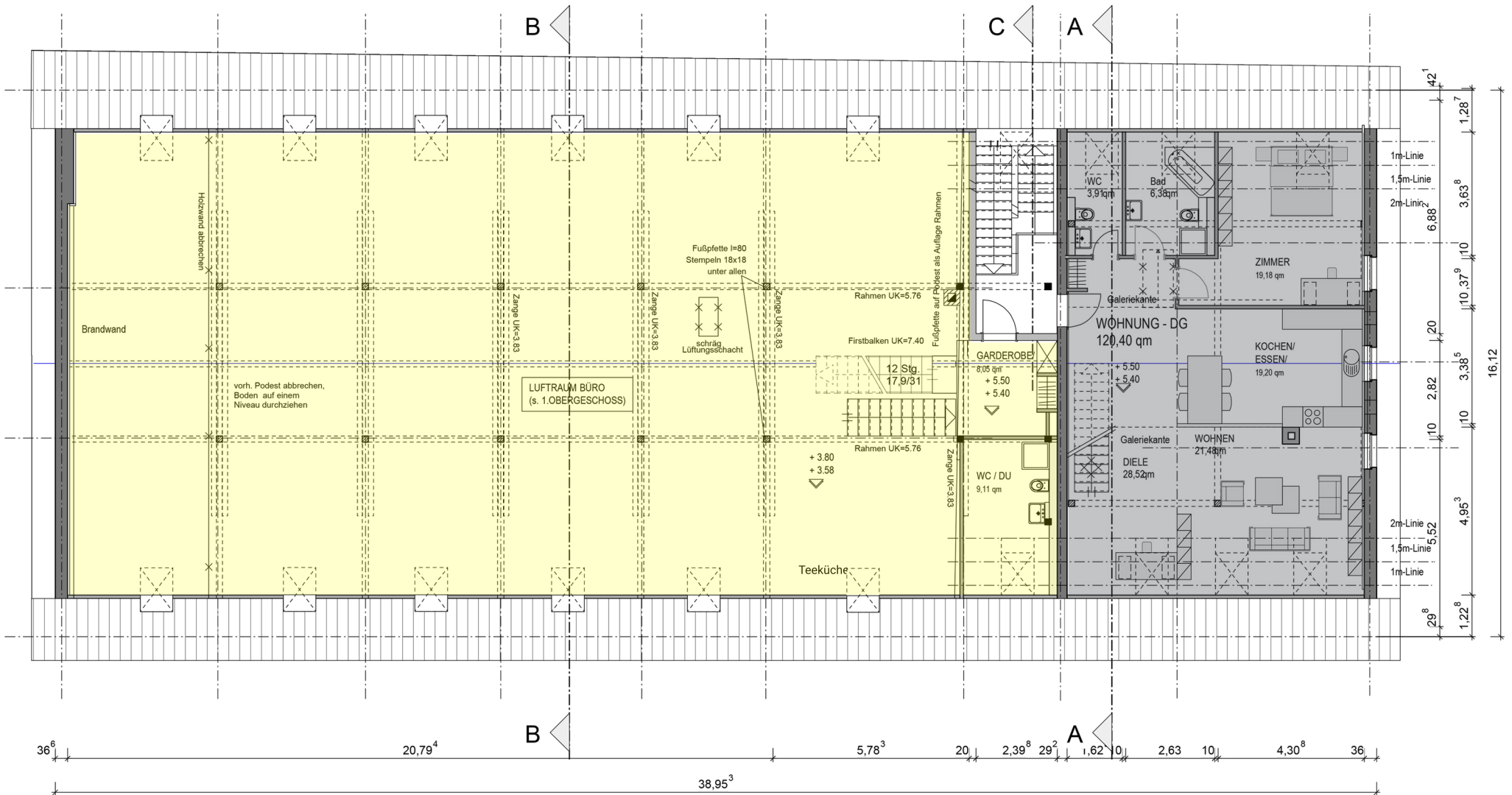
Grundriss Dachgeschoss M 1:100
