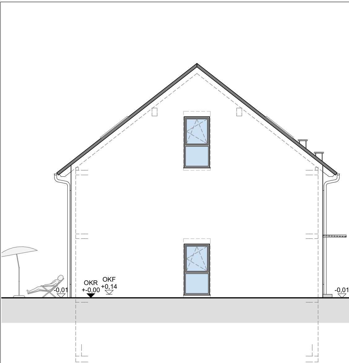
Giebelansicht
