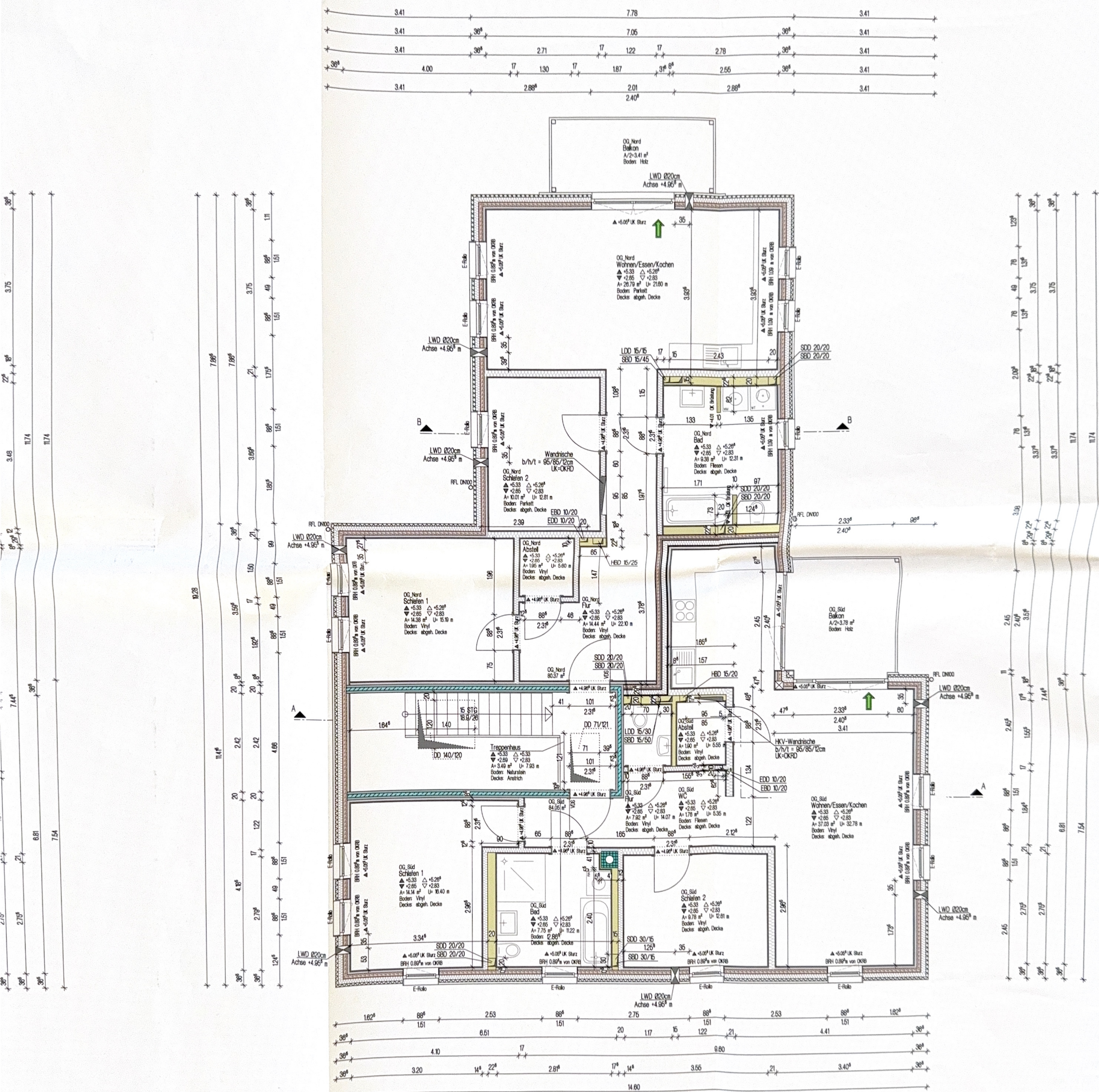
Grundriss Obergeschoss
