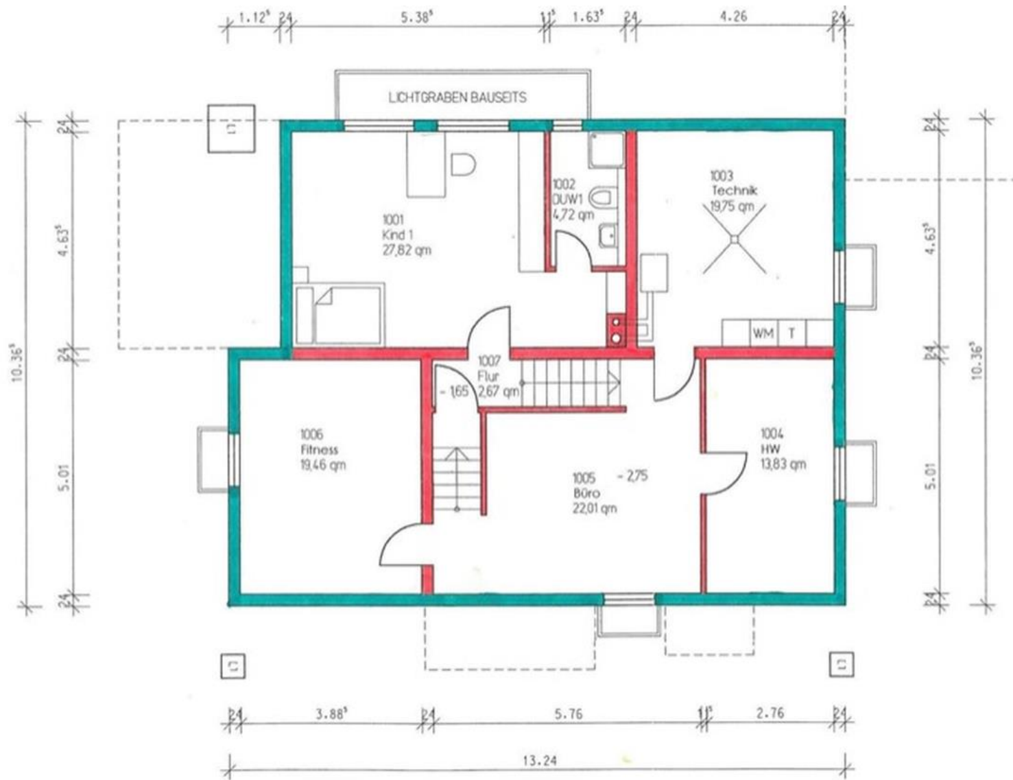
Untergeschoss
