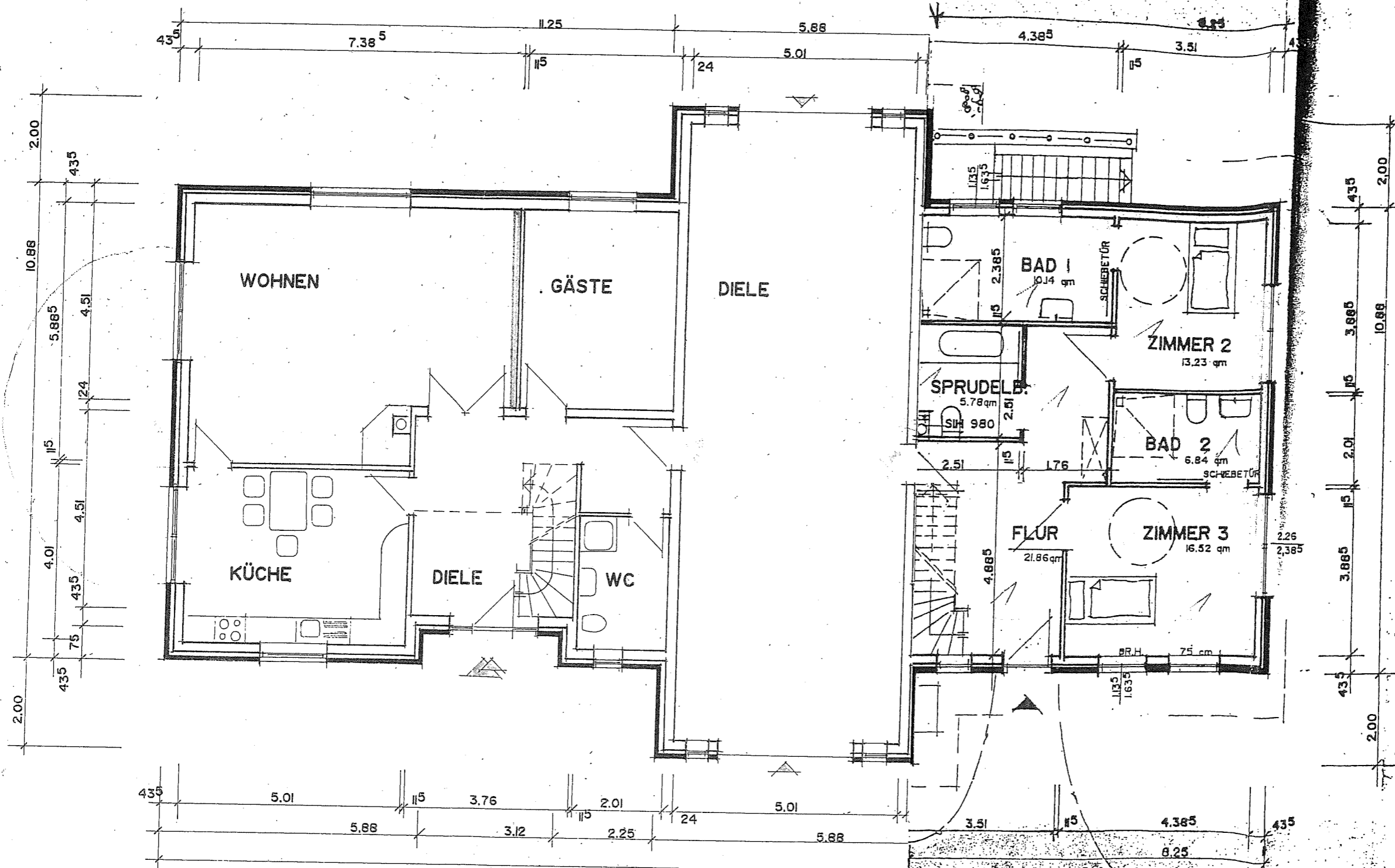
GRUNDRISS : ERDGESCHOSS , M. 1 : 100
