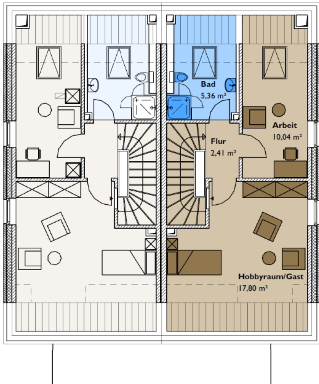
Dachgeschoss
