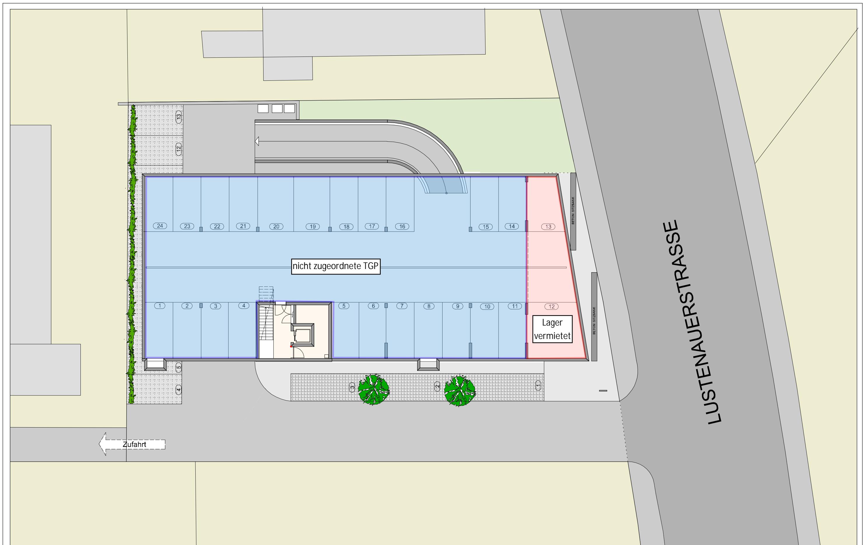
Büro- und Geschäftshaus "mono": Lustenauerstraße 56, 6850 Dornbirn UNTERGESCHOSS
