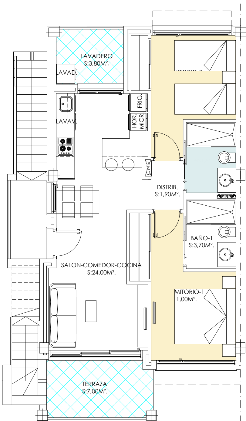
PLANTA PRIMERA
