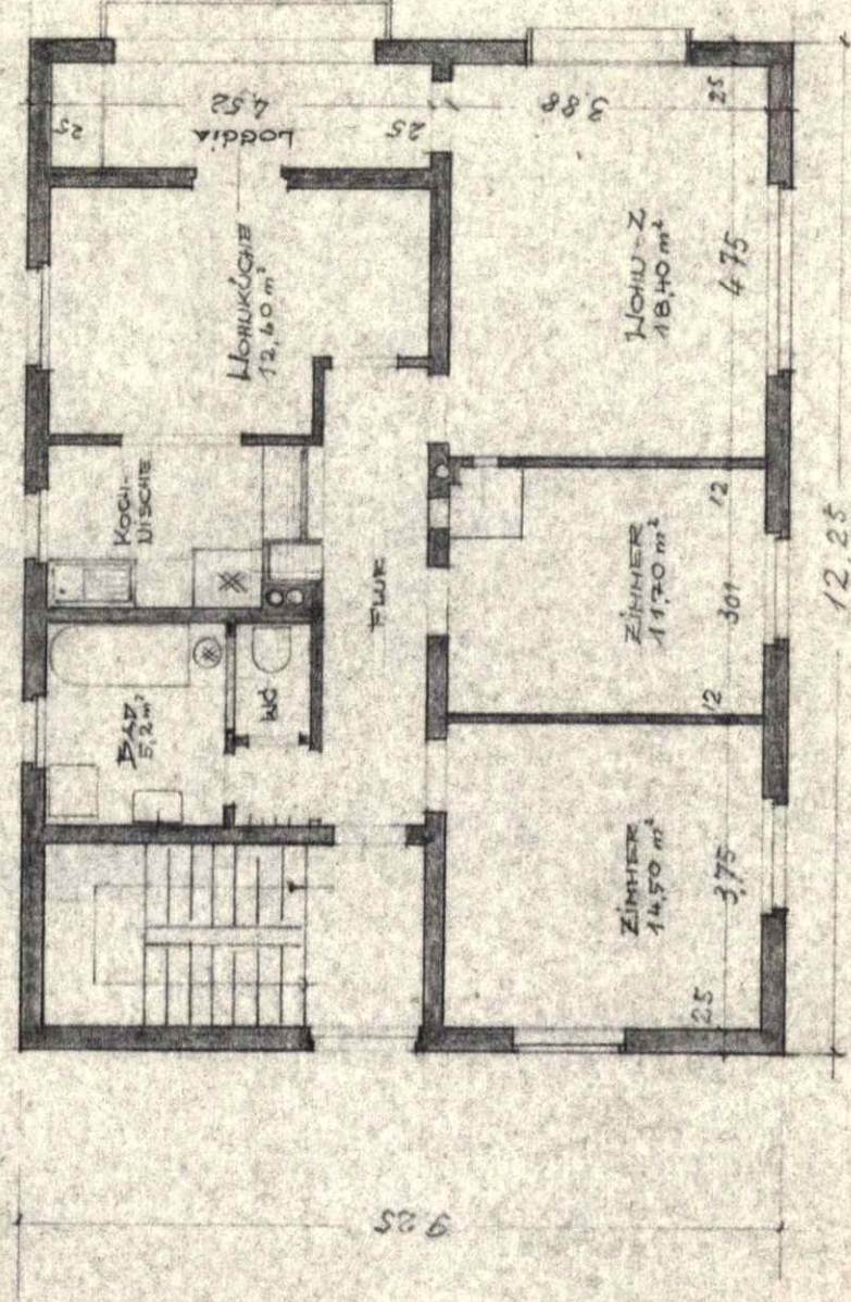
OBERGESCHOSS GRUNDRISS
