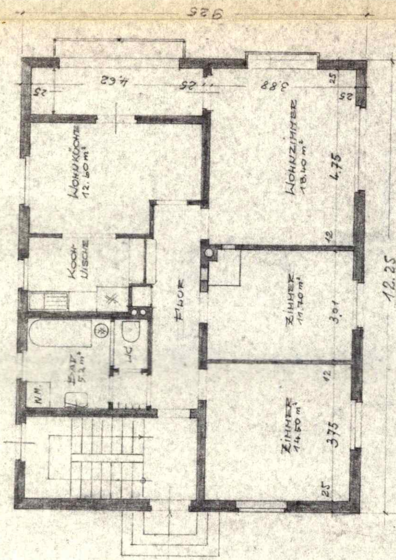
ERDGESCHOSS - GRUNDRISS
