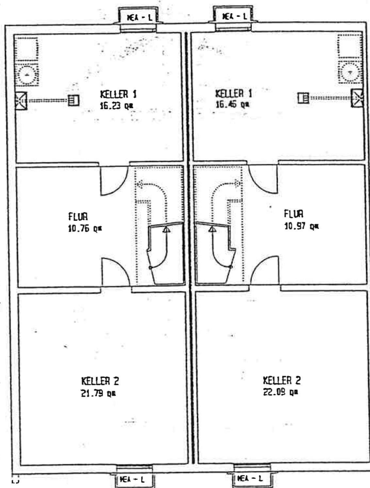
TYP '1' REIHEN-ENDHAUS
