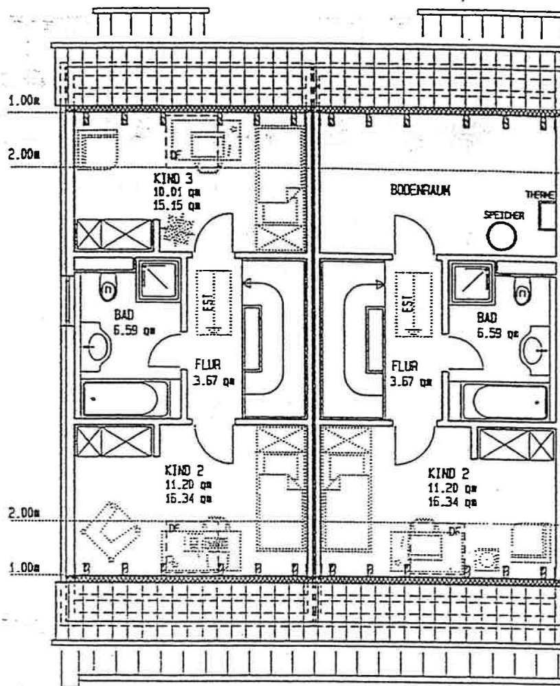
TYP '1' REIHEN-ENDHAUS
