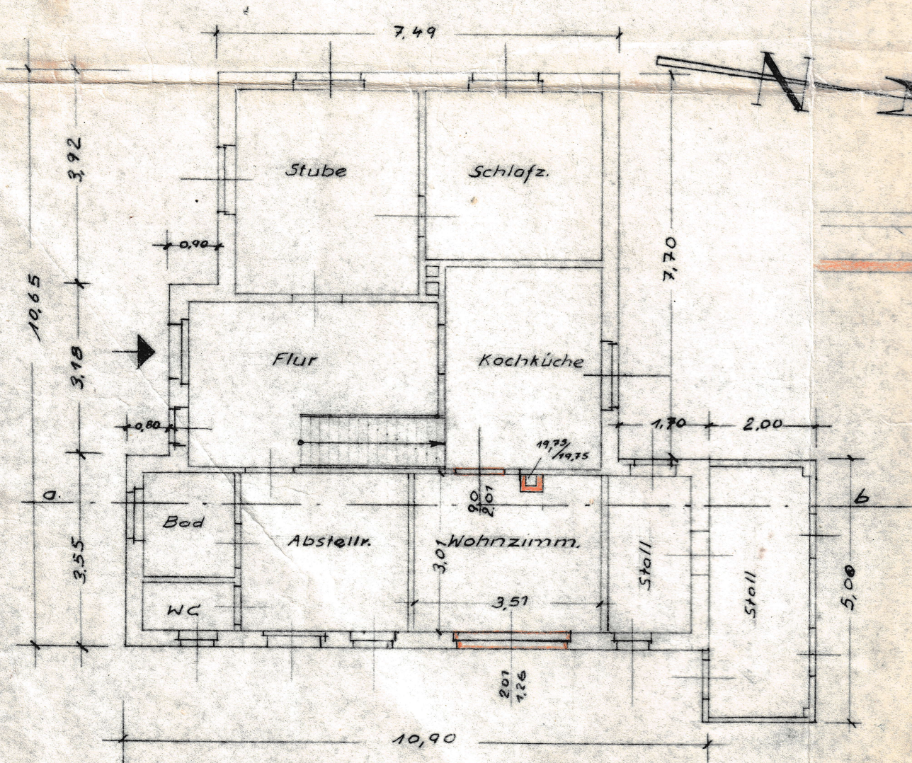
Erdgeschoss
