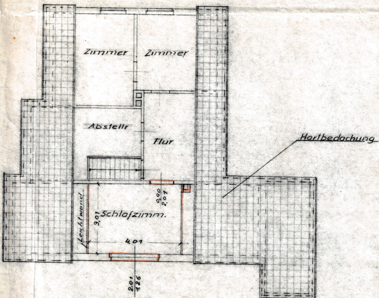
Dachgeschoss
