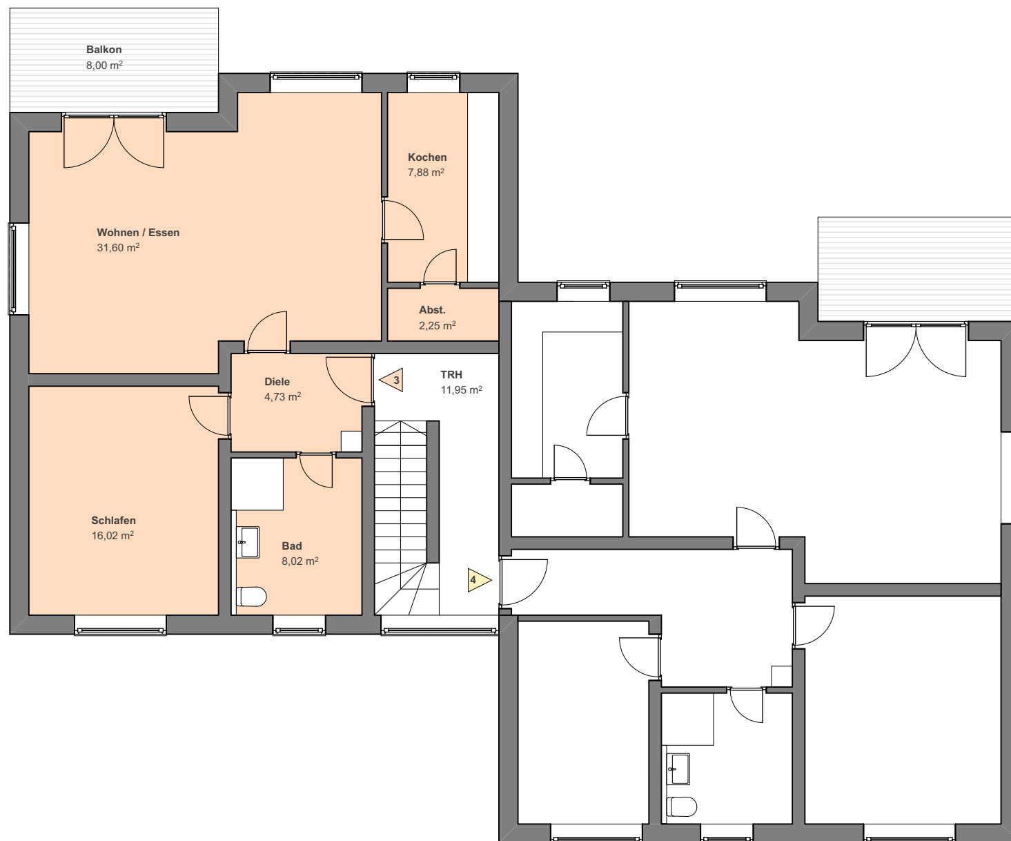
OBERGESCHOSS Wohnung 3
