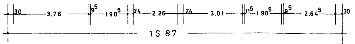
Erdgeschoss
